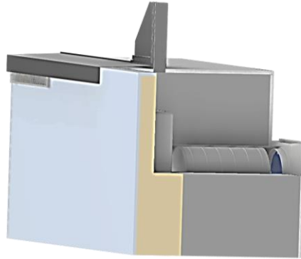
Unter Fensterbank - Außenansicht
