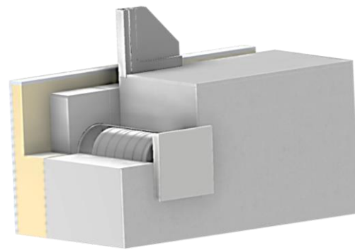
Horizontaler Verzug - Innenansicht
